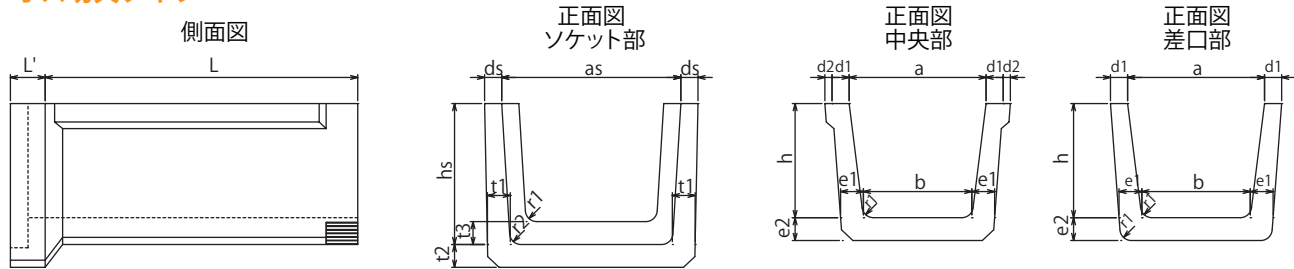
オス切欠タイプ・ベンチフリュームII型
