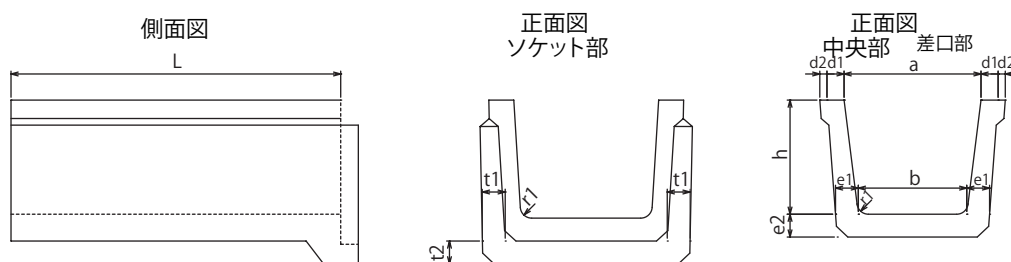
メス切欠タイプ・ベンチフリュームII型
