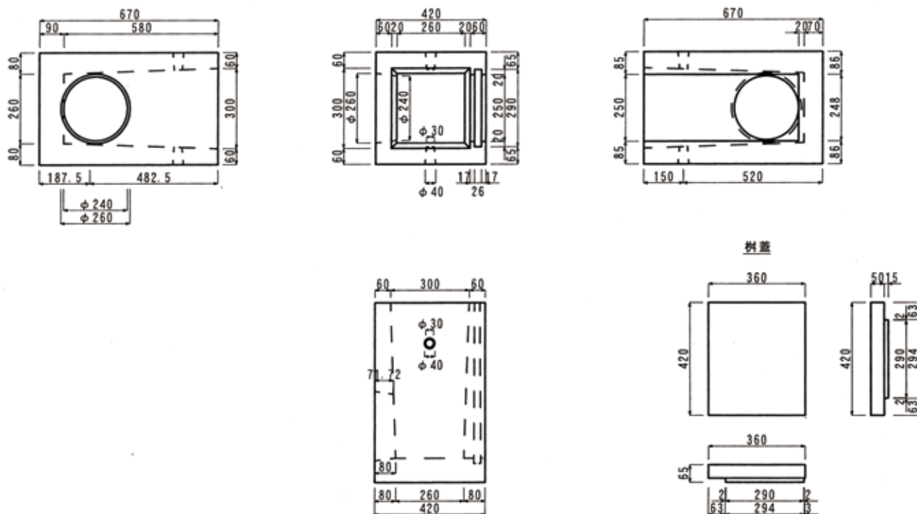
水路用組立柵 S型 田面排水柵の寸法表
